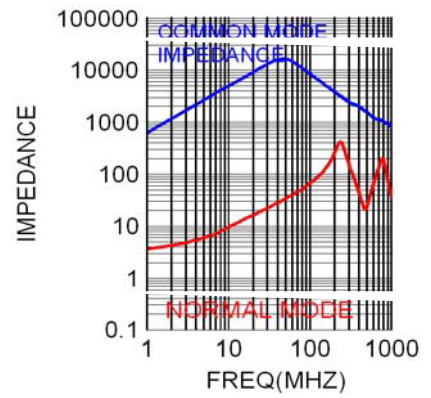
WCM-3225AUTOG-101YT01
