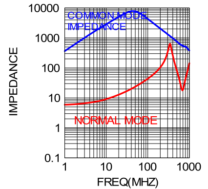
WCM-4532AUTO-510YT
