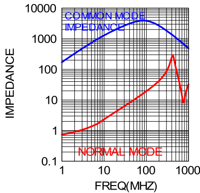
WCM-4532AUTO-220YT
