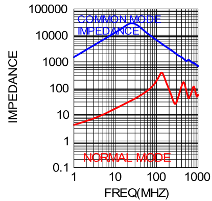
WCM-4532AUTO-201YT13
