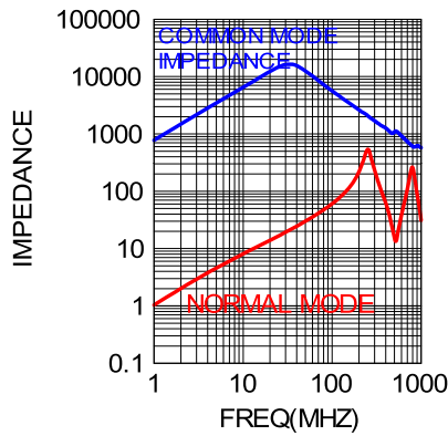
WCM-4532AUTO-101YT
